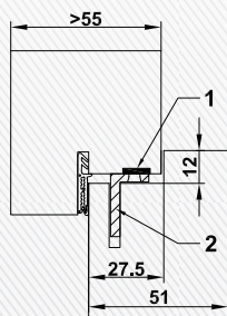
CombiModul überfält Vertikal- und Horizontalschnitt Oberblende - Rahmen
