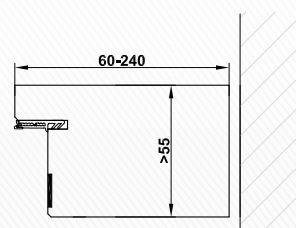
CombiModul Blockrahmen mit Rahmenverbreiterung
