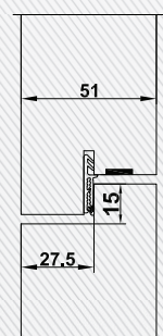
Vertikalschnitt Türblatt / Oberblende überfält
