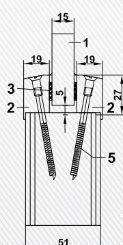
ohne Auskantung
