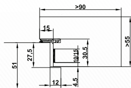
CombiModul-Blendrahmen
