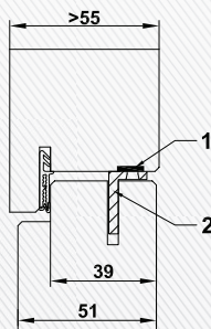
CombiModul stumpf Vertikal- und Horizontalschnitt Oberblende - Rahmen
