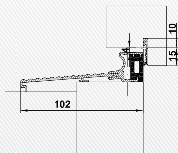
Typ H5, mit Thermoschwellen HEBGO 178 (mit Schwellenholz Eiche)
