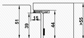
CombiModul stumpf Horizontalschnitt Türblatt - Rahmen
