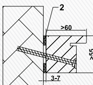
Blockrahmen MBW CombiModul mit Brandschutzacryl /-silikon
