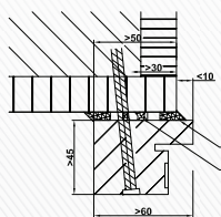
Blendrahmen CombiModul red. Querschnitt auf Holz-Ständerwand
