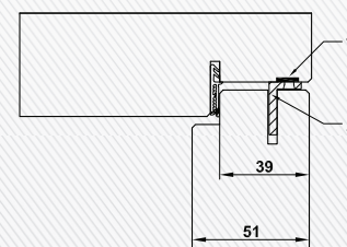
BLOCTool Vertikal- und Horizontalschnitt Oberblende - Rahmen
