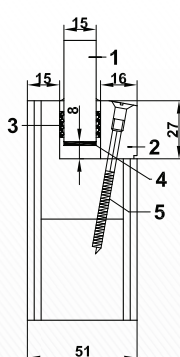
mit Auskantung
