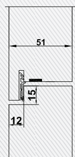
Vertikalschnitt Türblatt / Oberblende stumpf
