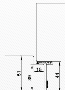
BLOCTool Horizontalschnitt Türblatt - Rahmen
