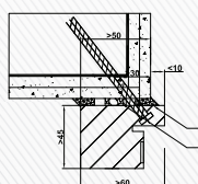
Blendrahmen LBW reduzierter Querschnitt
