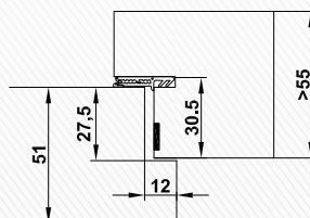
CombiModul überfält Horizontalschnitt Türblatt - Rahmen
