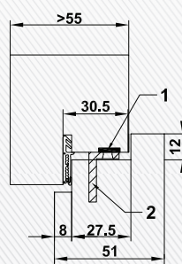
CombiModul überfält Vertikal- und Horizontalschnitt Oberblende - Rahmen
