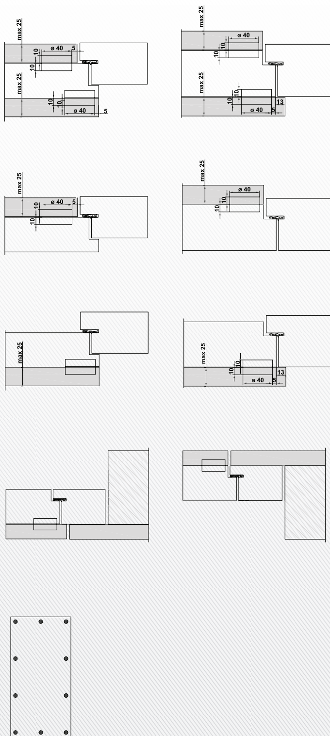
Anordnung Einhängebeschläge
