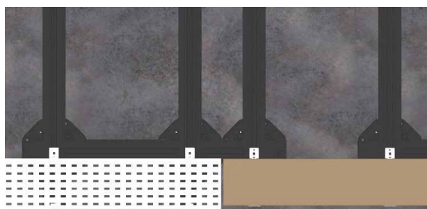
Bild 6. Das Drainageprofil ist 12 mm breiter als die WPC-Profile und der Abstand zur Gebäudewand sollte ca. 10 mm betragen.
