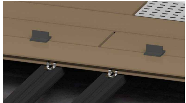
Bild 20. Mit Abstandhaltern kann einfach ein gleichmäßiges Fugenbild sichergestellt werden.
