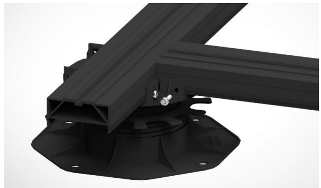
Bild 10. Die Querstücke müssen mit je 1 Bohrschraube 3,9 x 25 mm an dem Terrassenlager verschraubt werden.
