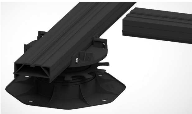
Bild 9. Wenn die ersten 2 Unterkonstruktionen aufgestellt sind, können ca. 336 mm lange Querstücke montiert werden.
