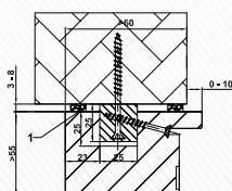
Blendrahmen MBW mit Montageleiste Hartholz
