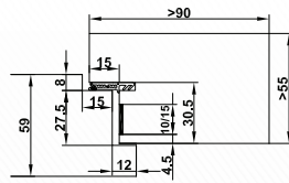
CombiModul-Blendrahmen Reduzierte Falztiefe 1-flg ohne Glas B_{\max} = 1030\text{mm} ; H_{\max} = 2200\text{mm}
