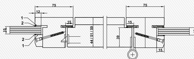
Ausführungsbeispiel Horizontalschnitt Pfosten -Türblatt
