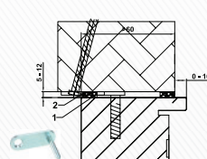
Blendrahmen MBW mit Z-Winkeln
