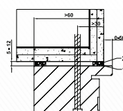
Blendrahmen LBW CombiModul
