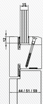
Ausführungsbeispiel Vertikalschnitt Türblatt - Kämpfer
