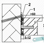
Blockrahmen MBW CombiModul mit Z-Winkel
