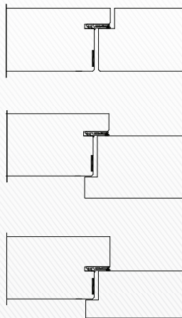
Beispiele Silencium VT - Tür
