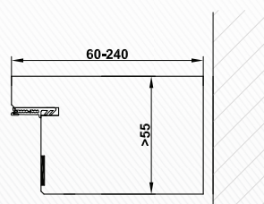
CombiModul Blockrahmen mit Rahmenverbreiterung
