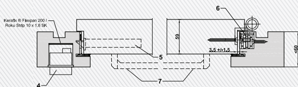
Horizontalschnitt CombiModul Blendrahmen
