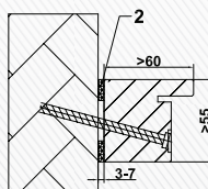
Blockrahmen MBW CombiModul mit Brandschutzacryl /-silikon
