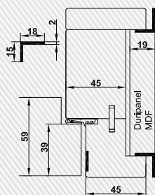
Blockfutter mit Futterbrett Alu-Winkel BLOTool BL
