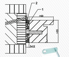
Blockrahmen CombiModul mit Z-Winkeln auf Holz-Ständerwand
