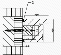
Blockrahmen CombiModul mit Montageleiste Hartholz auf Holz-Ständerwand
