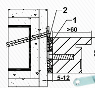
Blockrahmen LBW CombiModul mit Z-Winkel
