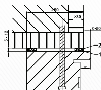
Blendrahmen CombiModul auf Holz-Ständerwand
