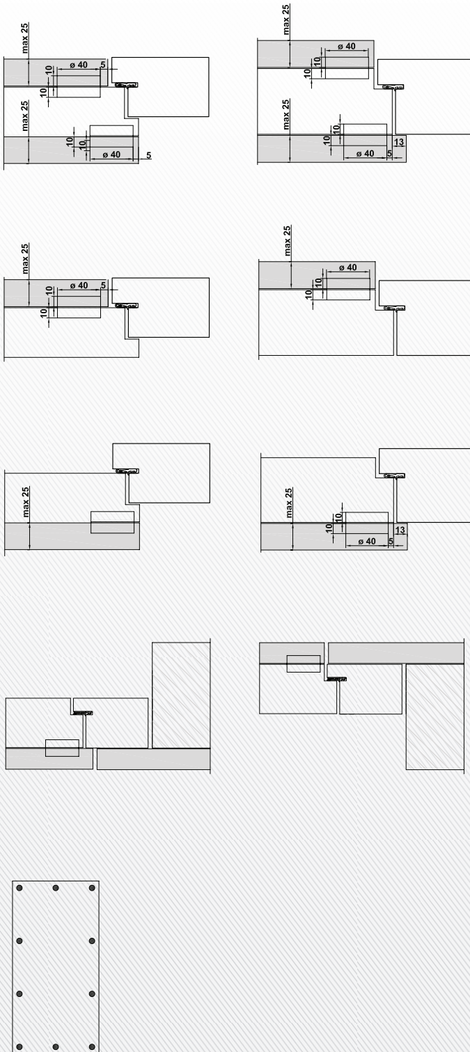
Anordnung Einhängebeschläge
