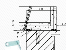
Blendrahmen LBW mit Z-Winkeln
