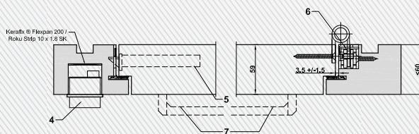
Horizontalschnitt CombiModul Blendrahmen
