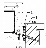
Blockrahmen LBW CombiModul, Rahmen überstehend
