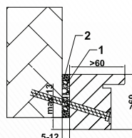
Blockrahmen MBW CombiModul, Rahmen überstehend
