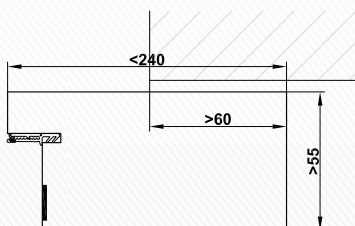
CombiModul Blendrahmen mit Rahmenverbreiterung
