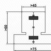
Pfosten / Kämpfer mit Kopplung
