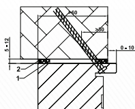
Blendrahmen MBW CombiModul
