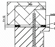
Blendrahmen MBW CombiModul
