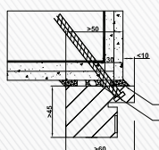
Blendrahmen LBW reduzierter Querschnitt
