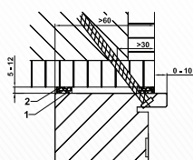
Blendrahmen CombiModul auf Holz-Ständerwand
