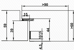
CombiModul-Blendrahmen
