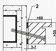
Blockrahmen LBW CombiModul mit Brandschutzacryl /-silikon
