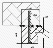
Blendrahmen MBW reduzierter Querschnitt
