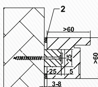
Blockrahmen MBW CombiModul mit Montageleiste Hartholz
