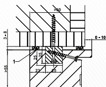
Blendrahmen CombiModul mit Montageleiste Hartholz auf Holz-Ständerwand
