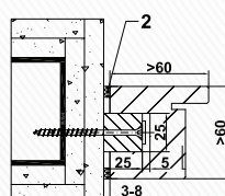
Blockrahmen LBW CombiModul mit Montageleiste Hartholz
