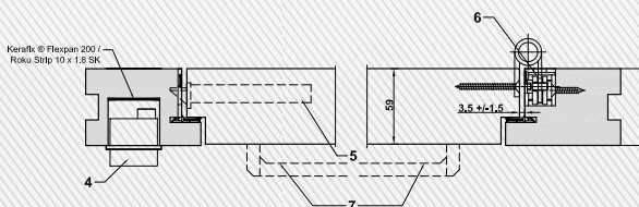
Horizontalschnitt CombiModul Blockrahmen
