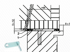
Blendrahmen CombiModul mit Z-Winkeln auf Holz-Ständerwand
