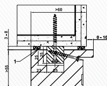
Blendrahmen LBW mit Montageleiste Hartholz
