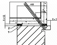
Blendrahmen LBW CombiModul
