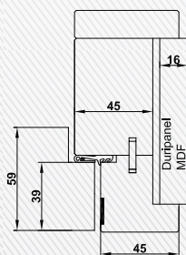
Blockfutter mit Futterbrett BLOTool BL
