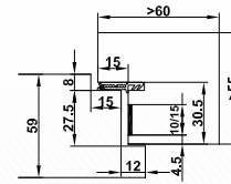
CombiModul-Blockrahmen Reduzierte Falztiefe 1-flg ohne Glas B_{\max} = 1030\text{mm} ; H_{\max} = 2200\text{mm}
