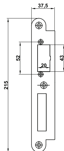
BRUNEX® E-Öffner Flachschliessblech für überfälzte und stumpfeinschlagende Türen
