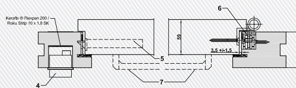
Horizontalschnitt CombiModul Blockrahmen
