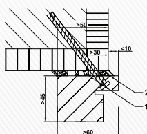
Blendrahmen CombiModul red. Querschnitt auf Holz-Ständerwand
