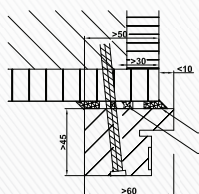
Blendrahmen CombiModul red. Querschnitt auf Holz-Ständerwand
