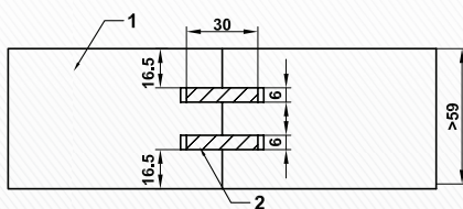
Kopplung Trennwand-Elemente
